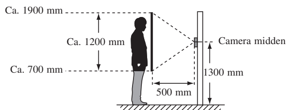
Montagepositie 1300 mm
